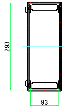
A-A ( 1 : 6.5 )
